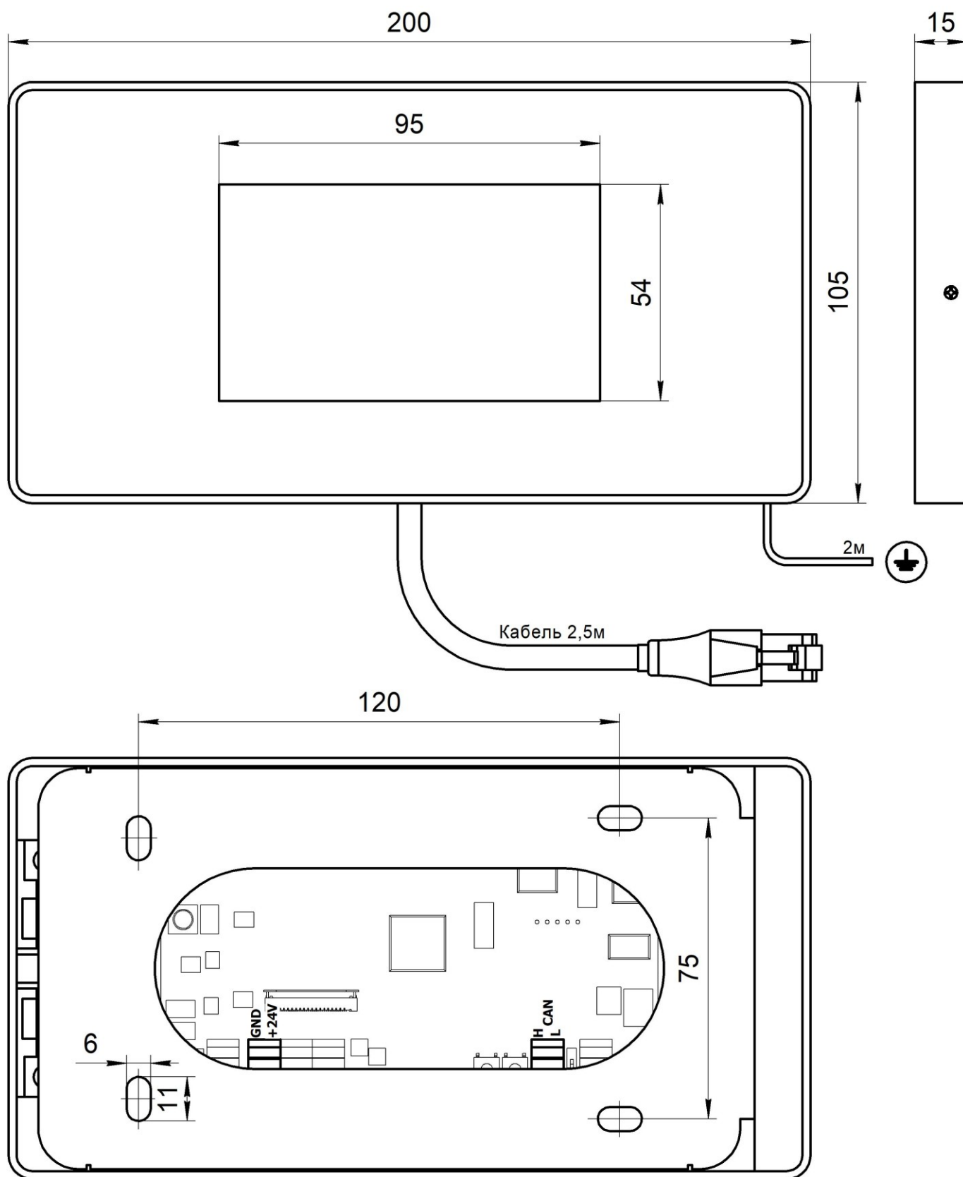
Рис.1 Внешний вид Табло накладное ОНИКС (жгут RJ45) НШЕК.468232.138
